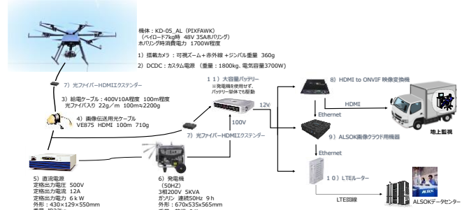
有線ドローンを用いた広域監視システム
